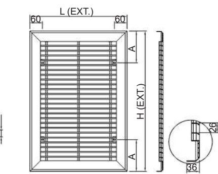
RPK-P REJILLA FIJA Y TORNILLOS OCULTOS
