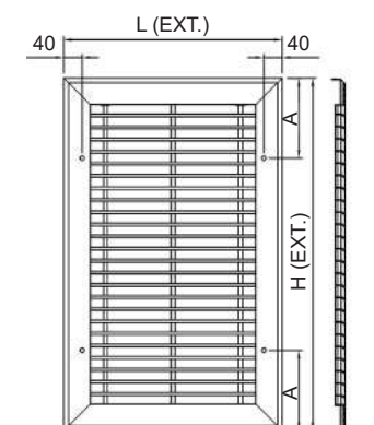
RPK REJILLA FIJA Y TORNILLOS VISTOS
