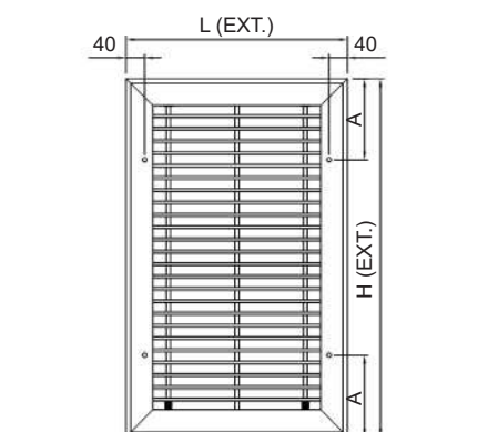
RPK-1A REJILLA DESMONTABLE Y TORNILLOS VISTOS
