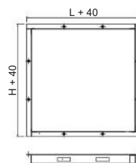
Marco metálico para 210-TA
