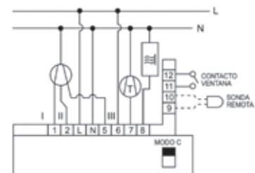
ESQUEMA 4: Bomba de calor con maniobra sobre compresor y válvula inversora energizada en calor. La válvula está permanentemente energizada cuando se selecciona el funcionamiento en calor.
